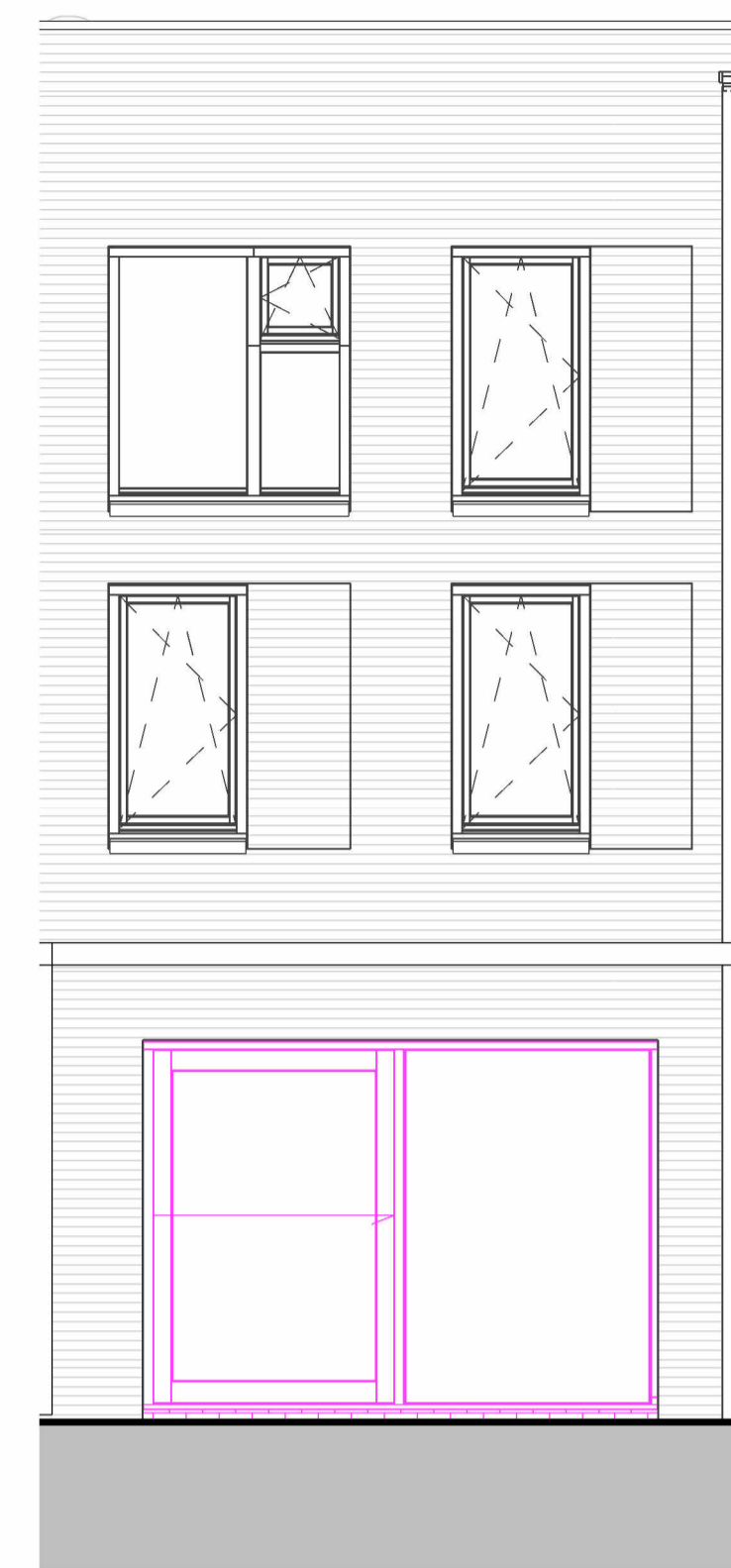
A3-202: bredere schuifpui achtergevel circa 3,4m
