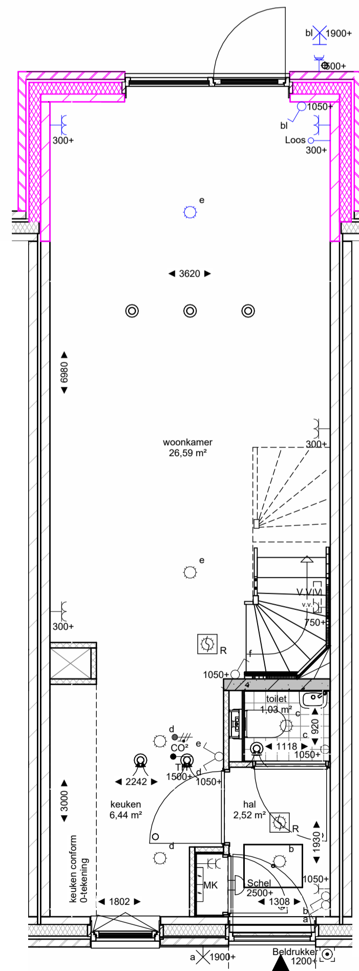
A1-180: Uitbouw 1,8m achtergevel
