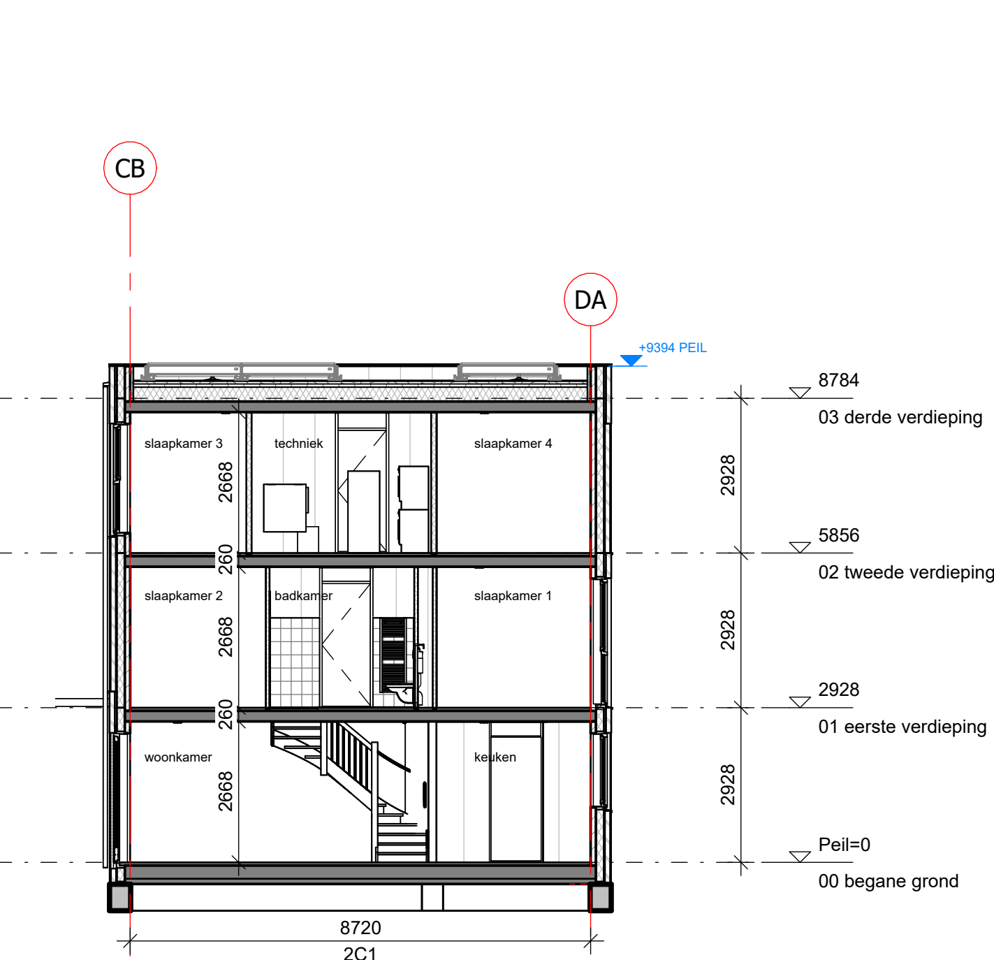
doorsnede D-D
