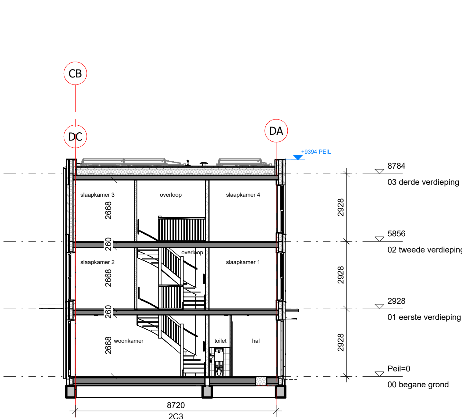
doorsnede C-C
