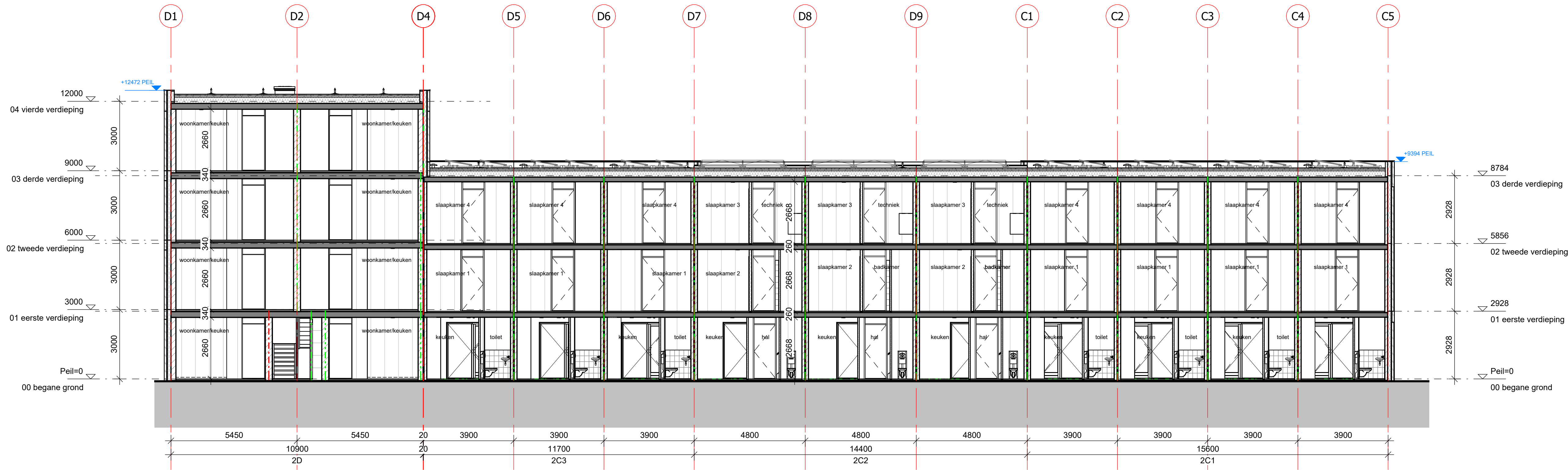
doorsnede A-A
