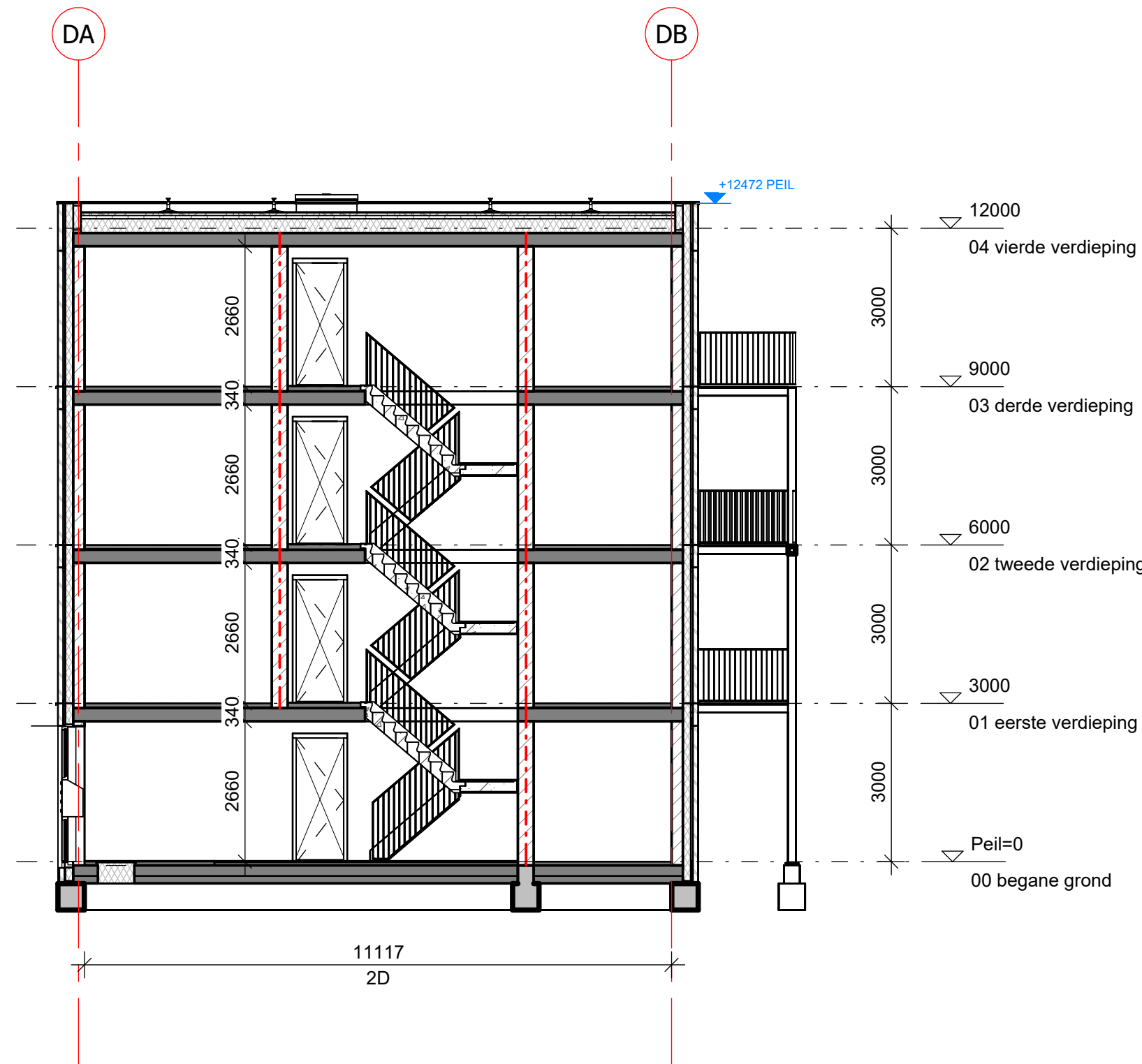
doorsnede E-E
