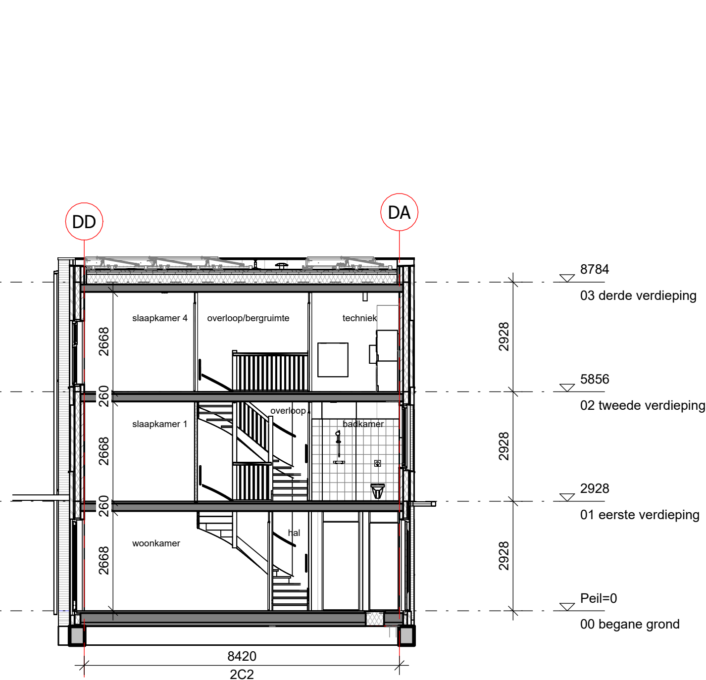
doorsnede B-B
