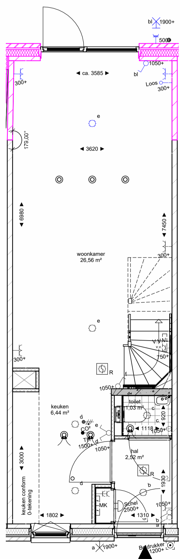
bnr 178 A1-180: Uitbouw 1,8m achtergevel
