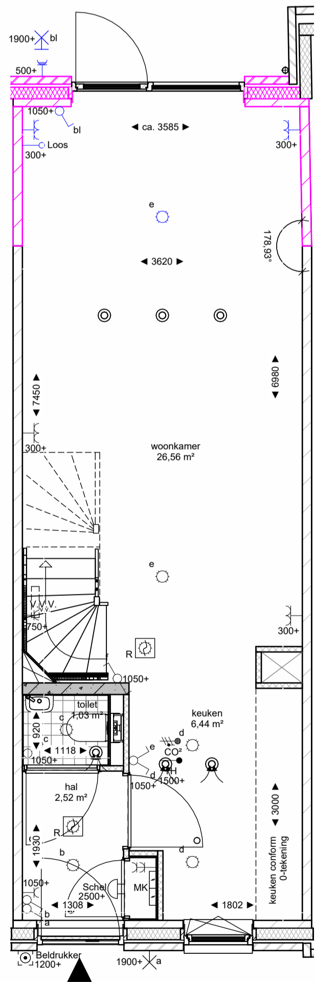
bnr 176 A1-180: Uitbouw 1,8m achtergevel
