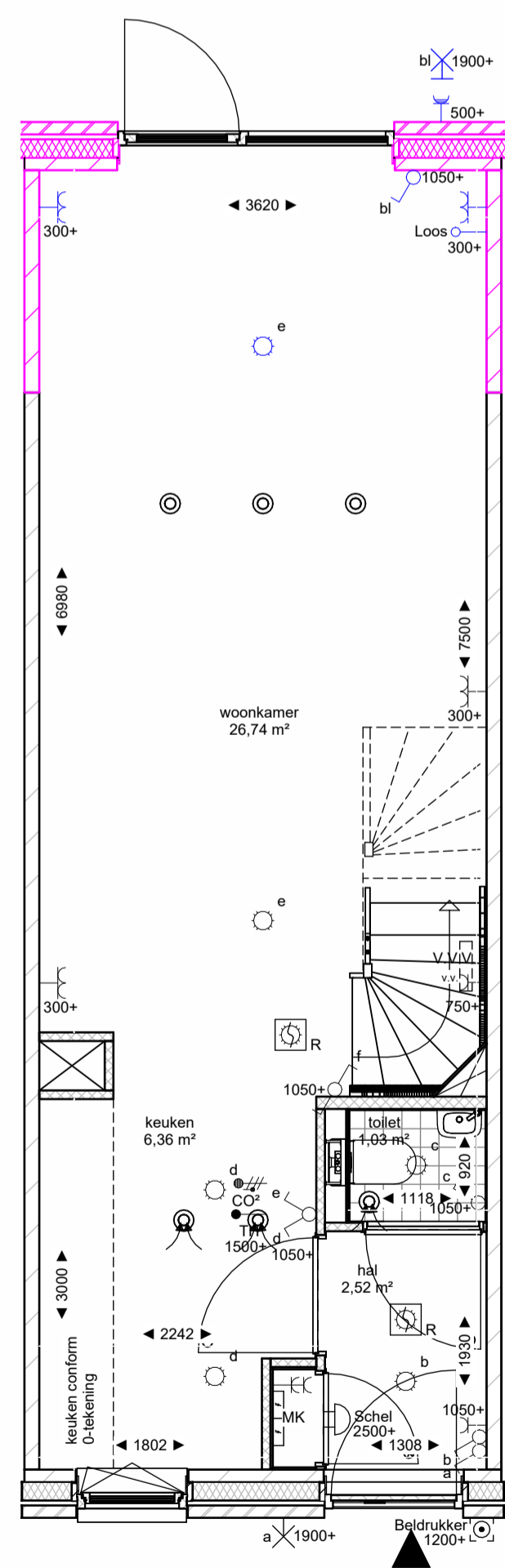
bnr 177 A1-180: Uitbouw 1,8m achtergevel
